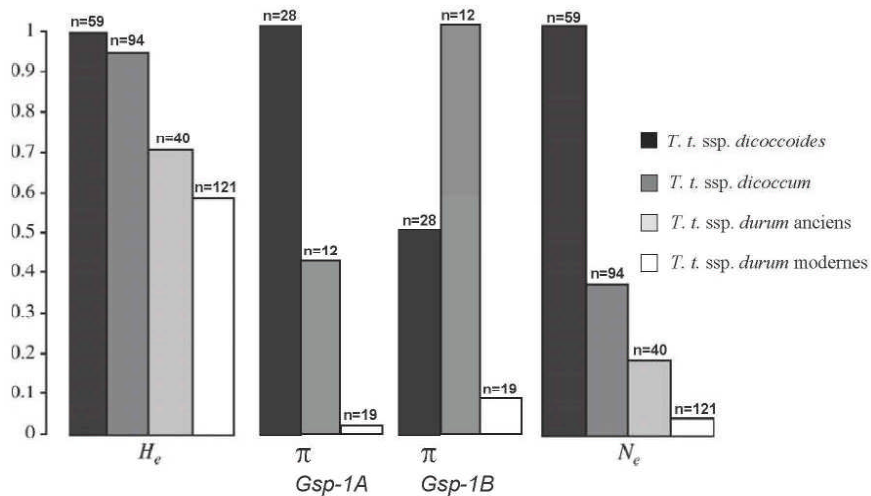
Figure 3 : Comparaison des patrons de diversité dans différents compartiments du complexe de Triticum turgidum . Les hétérozygoties de Nei ( H_e ) de chaque compartiment, moyennes sur 15 locus microsatellites sont exprimées en valeur relative par rapport à la diversité moyenne observée chez le groupe « dicoccoides ». Au milieu les patrons de diversité nucléotidique chez les deux copies homéologues du gène Gsp-1 (copie A et B) sont comparées en utilisant l'hétérozygotie moyenne des sites ( \pi ). A droite les tailles efficaces ( N_e ) relatives, estimées en utilisant le polymorphisme microsatellites de chaque compartiment sont données. Pour l'analyse du polymorphisme des Gsp-1 , les blés durs anciens et modernes sont regroupés.
