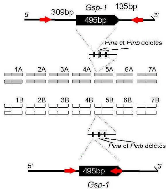
Figure 2 : Environnement génomique et structure des copies homéologues du gène Gsp-1 chez T. turgidum . Le gène Gsp-1 n'a pas d'intron et est d'une longueur de 495 bp. Les amorces utilisées pour amplifier de façon spécifique et séquencer chacune des deux copies homéologues du gène Gsp-1 (génomme A et génome B) sont représentées par des flèches rouges. NB : Les gènes de puroindolines ( Pina et Pinb ) sont absents dans les espèces tétraploïdes de génome AB alors qu'ils sont présents dans les espèces diploïdes progénitrices sauvages.
