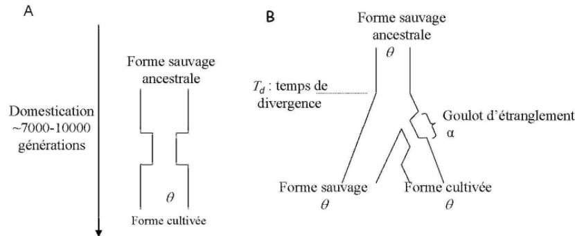
Figure 5: Représentation schématique des deux scénarios considérés pour étudier l'histoire évolutive de la luzerne cultivée. (A) Scénario représentant uniquement le goulot d'étranglement lié à la domestication (B) Scénario prenant en compte l'information obtenue sur le compartiment sauvage actuel. On considère ici que le compartiment sauvage est le descendant direct de la population sauvage dans laquelle la forme cultivée a été échantillonnée. \theta : taux de mutation efficace \alpha : intensité du goulot d'étranglement.
