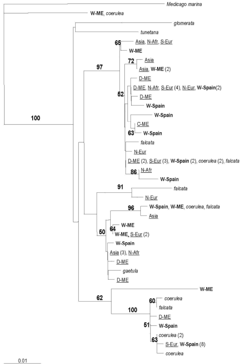
Figure 4 : Arbre (obtenu par la méthode dite du « neighbor-joining ») des différents haplotypes identifiés pour la région Pect . Les valeurs de bootstrap sont données en pourcentage lorsque la valeur excède 50 %. A côté de chaque haplotype est indiqué dans quel(s) groupe(s) l'haplotype a été identifié (le nombre entre parenthèse précise combien d'individus de ce groupe ont présenté cet haplotype (si ce nombre excède
